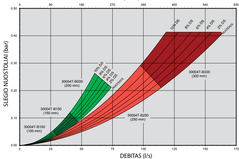
MODELIS „30004T“ DEBITAS (m³/h)
